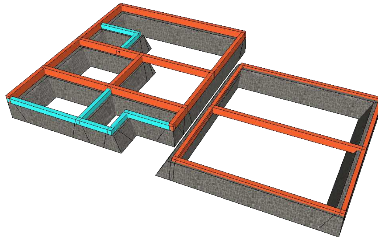
PERSPEKTIF PONDASI skala NTS
