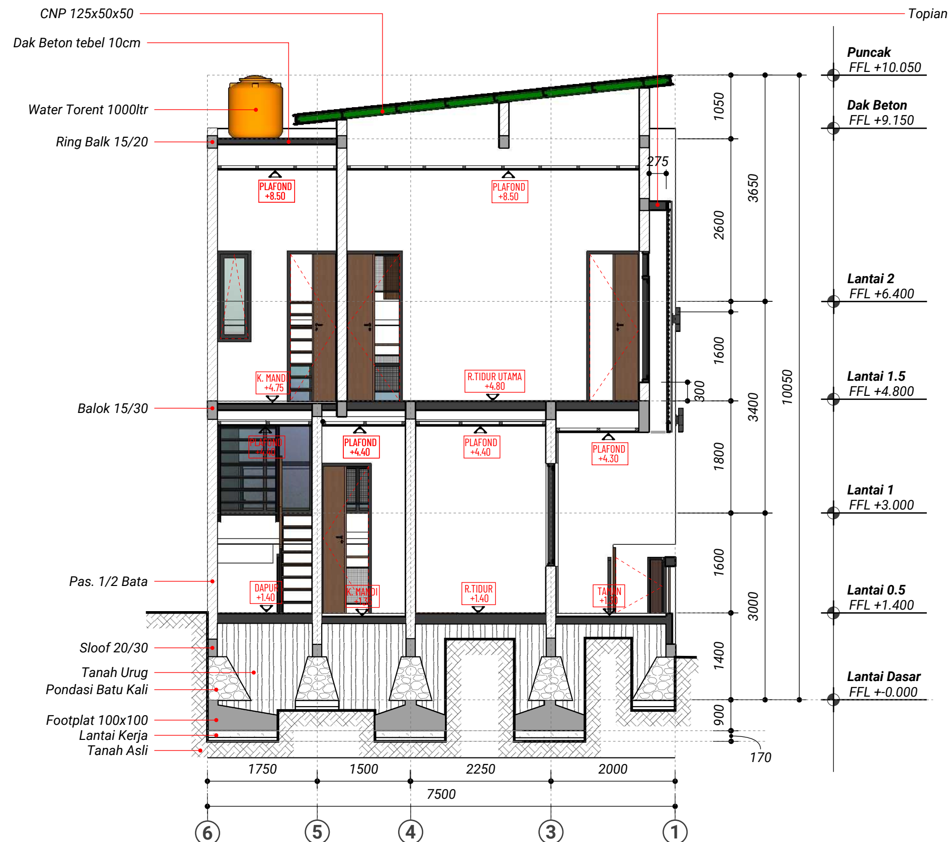
POTONGAN A-A skala 1 : 100
