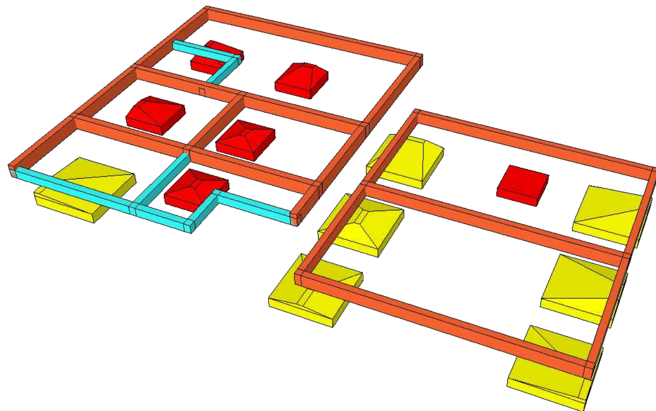
PERSPEKTIF FOOTPLAT & SLOOF skala NTS
