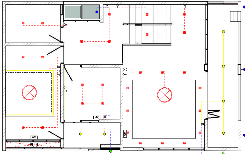
DENAH KELISTRIKAN LANTAI 2 skala 1 : 100
