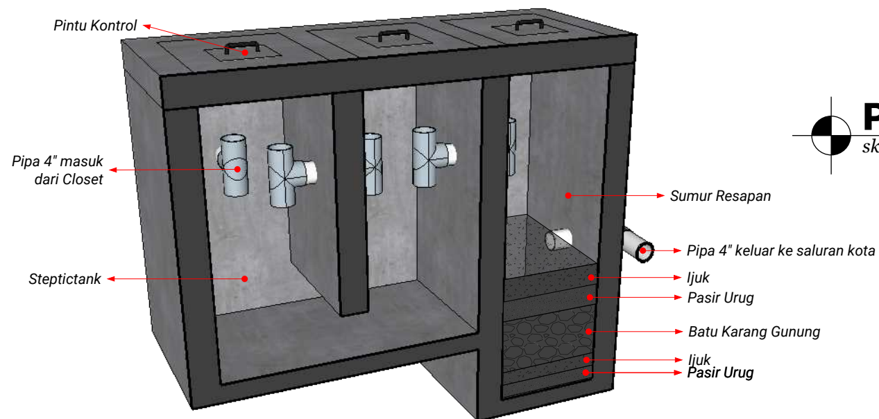
PERSPEKTIF STEPTICTANK skala 1 : NTS
