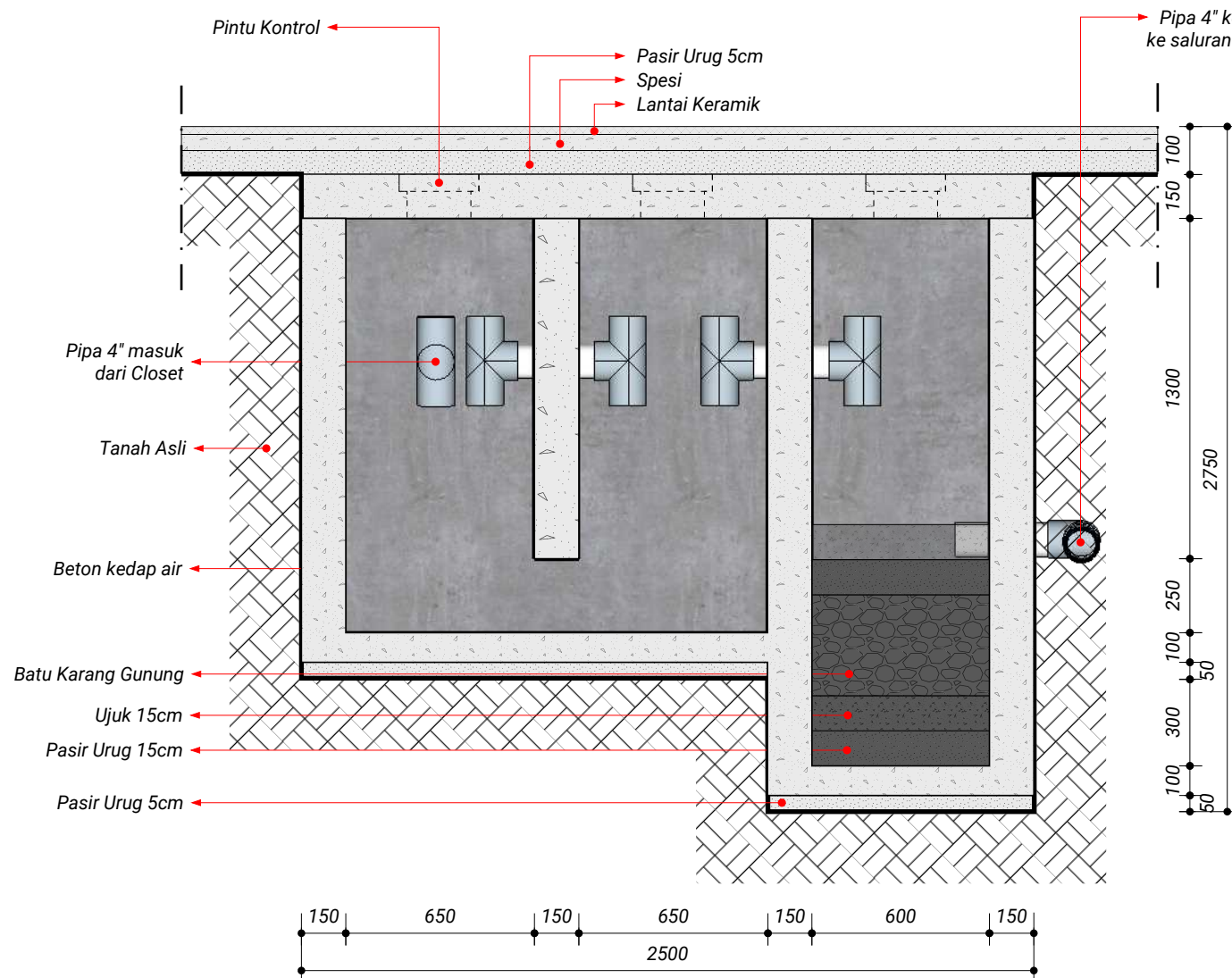
POTONGAN - A skala 1 : 50
