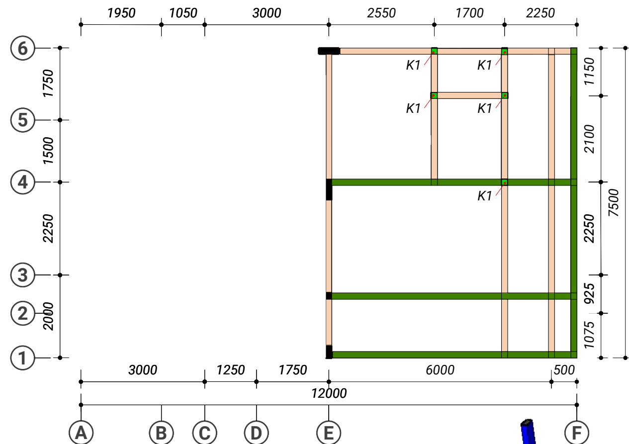
DENAH KOLOM LANTAI 2,5 skala 1 : 100
