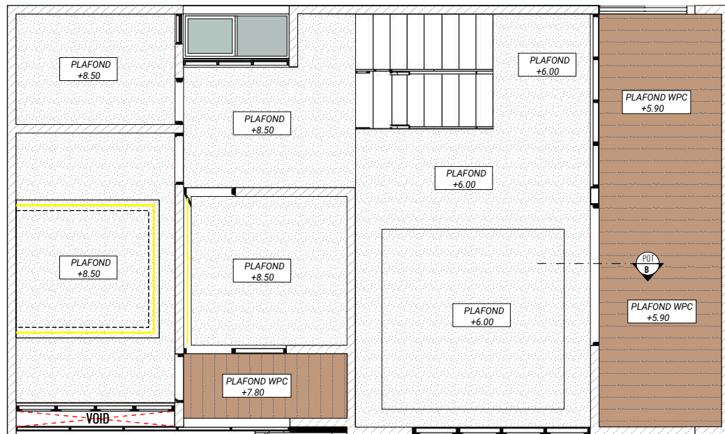
DENAH PLAFOND LANTAI 2 skala 1 : 100
