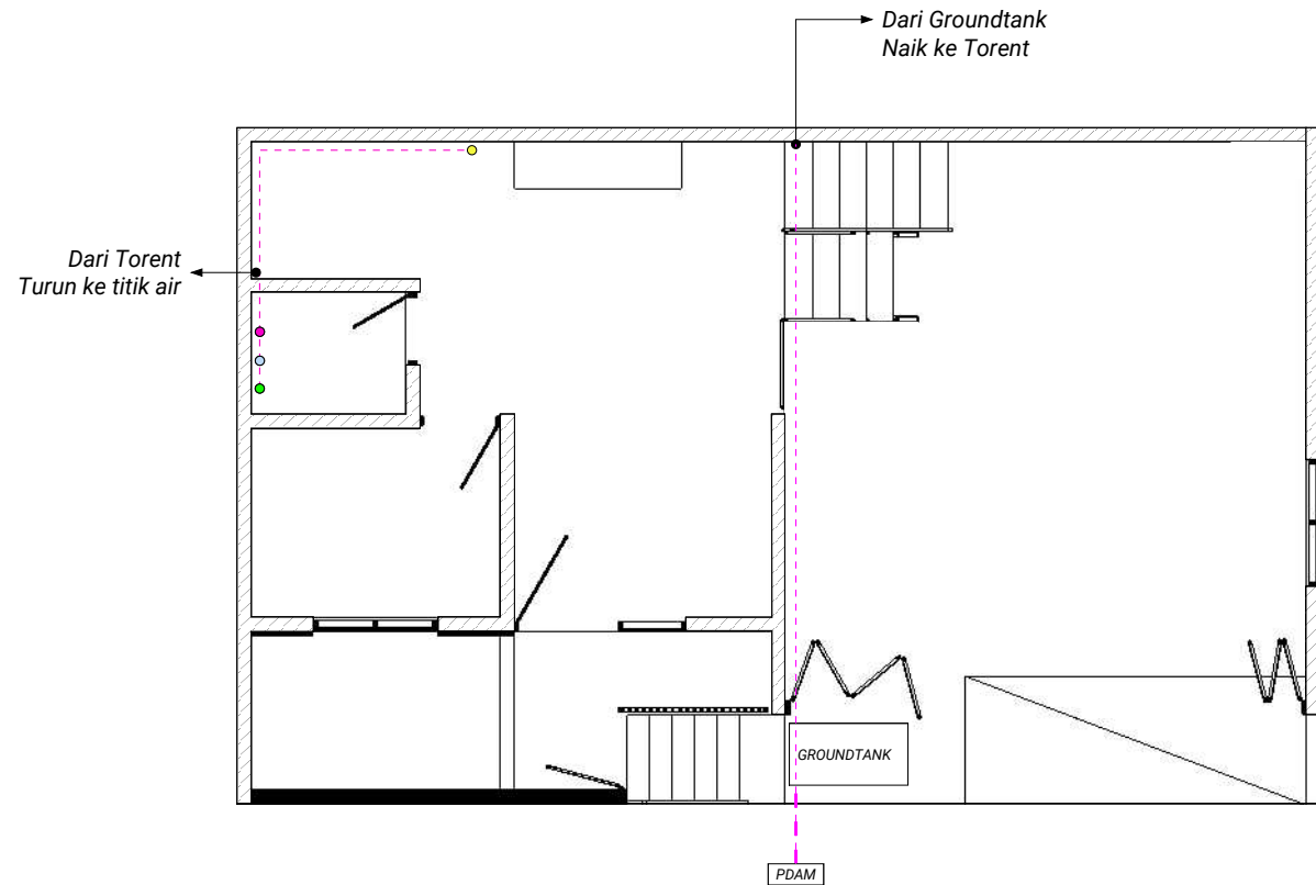
DENAH AIR BERSIH LANTAI 1 skala 1 : 100
