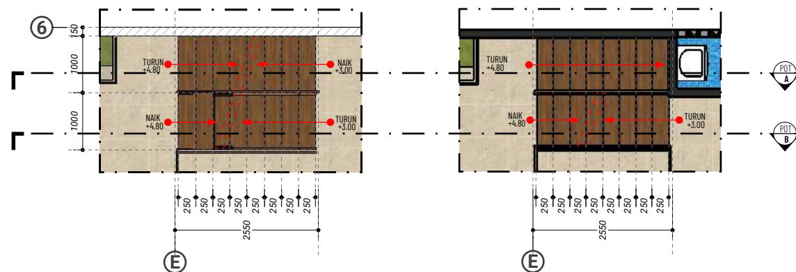
DENAH TANGGA skala 1 : 100
