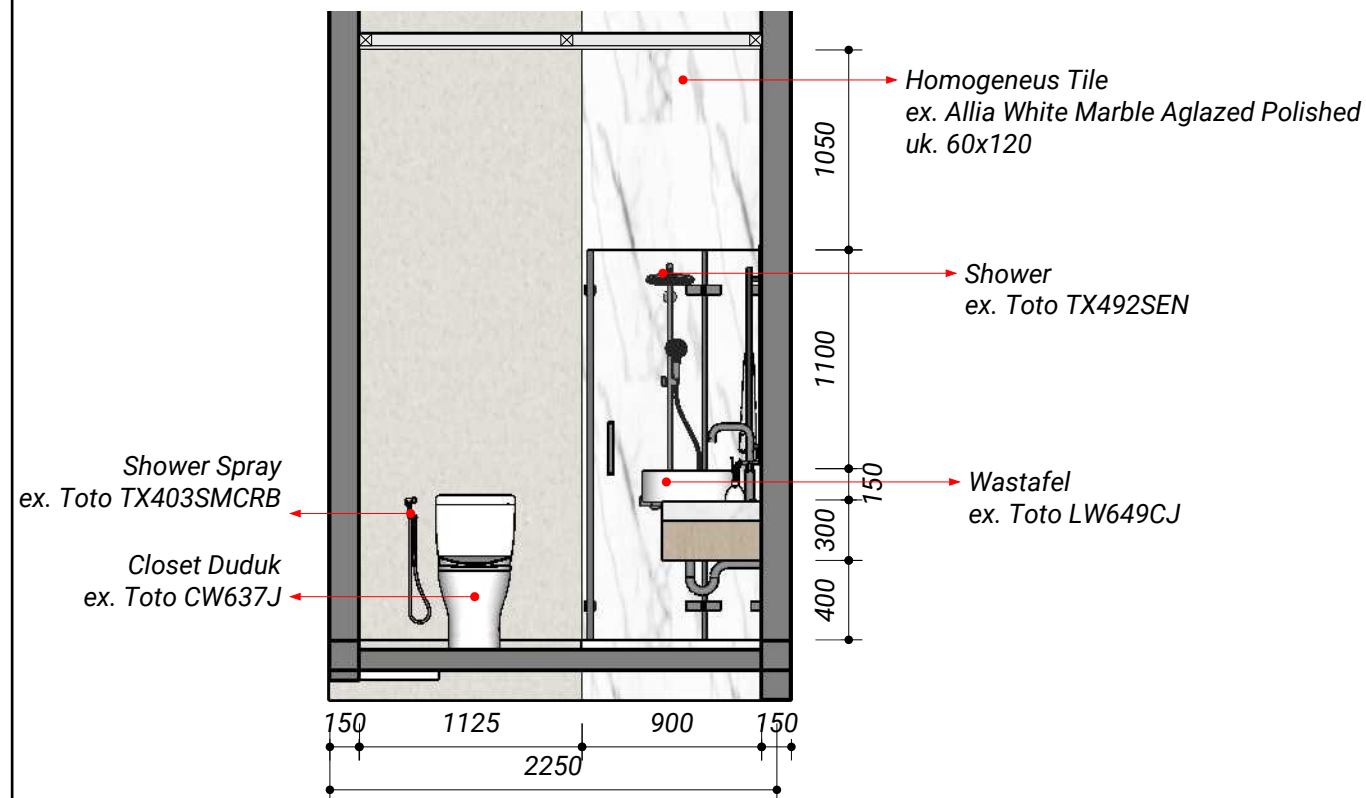
POTONGAN - A
