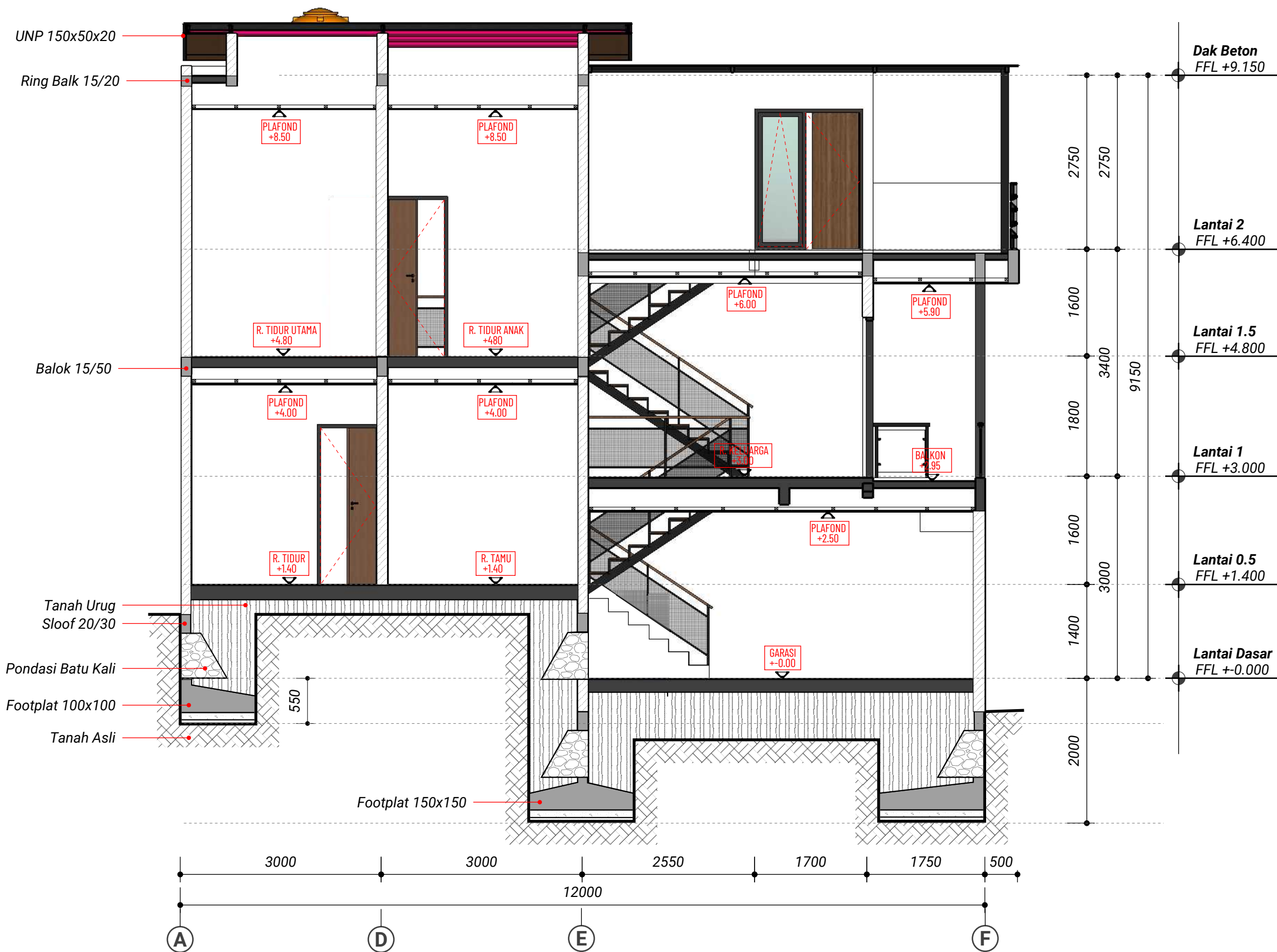
POTONGAN E-E skala 1 : 100
