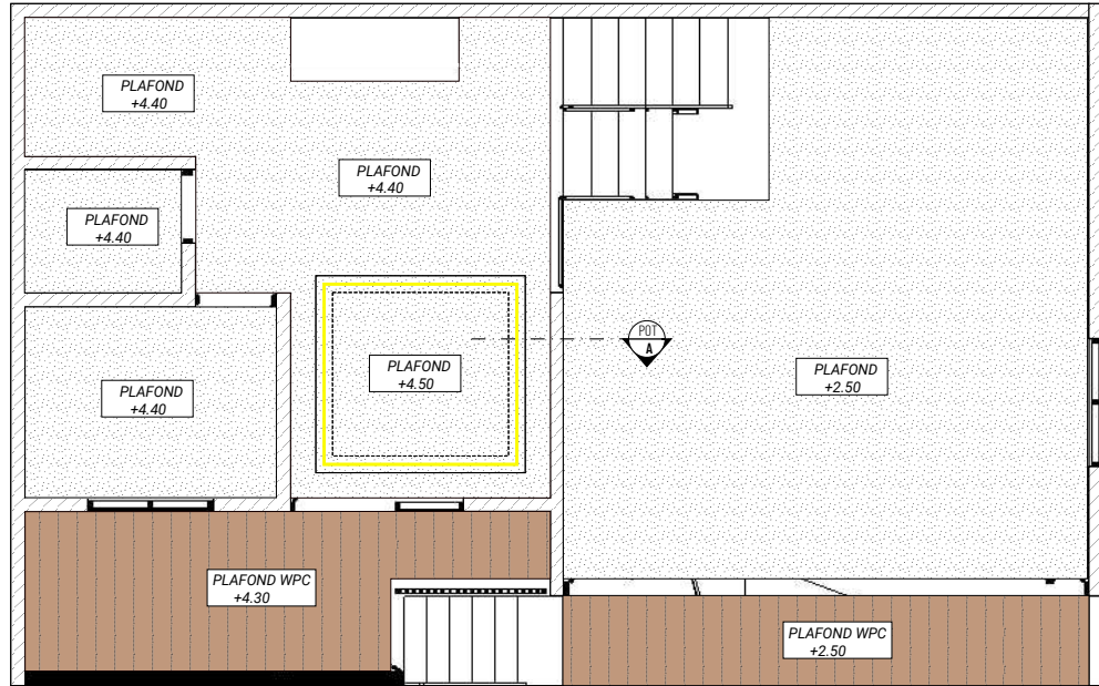
DENAH PLAFOND LANTAI 1 skala 1 : 100
