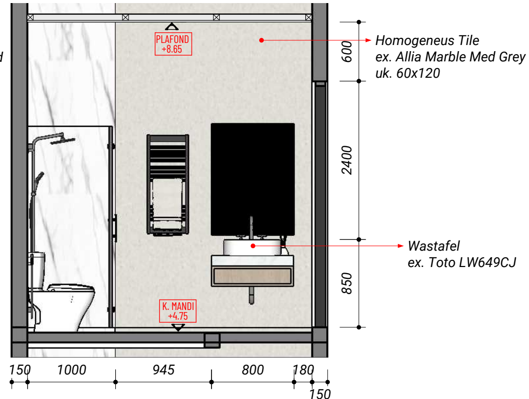
POTONGAN - B
