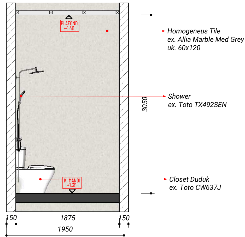
POTONGAN - B skala 1 : 50
