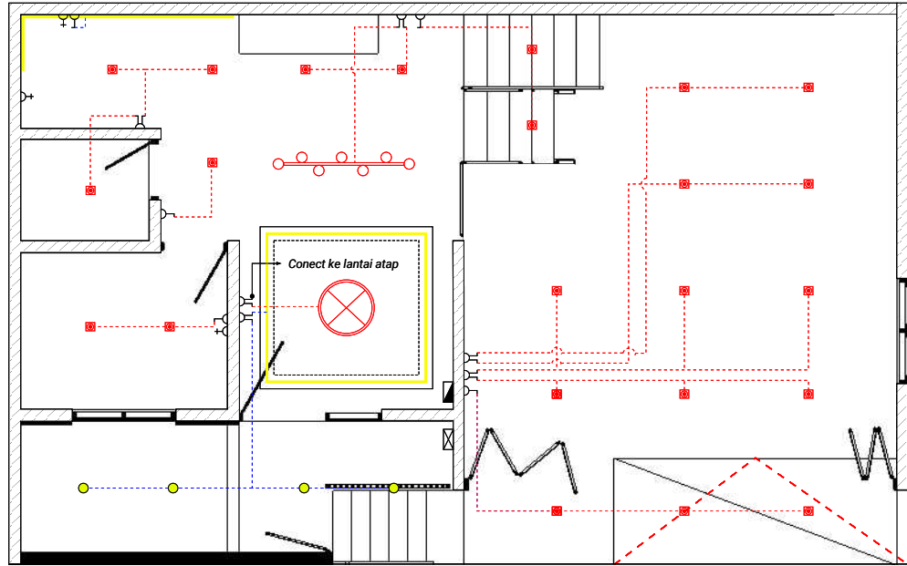
DENAH KELISTRIKAN LANTAI 1 skala 1 : 100
