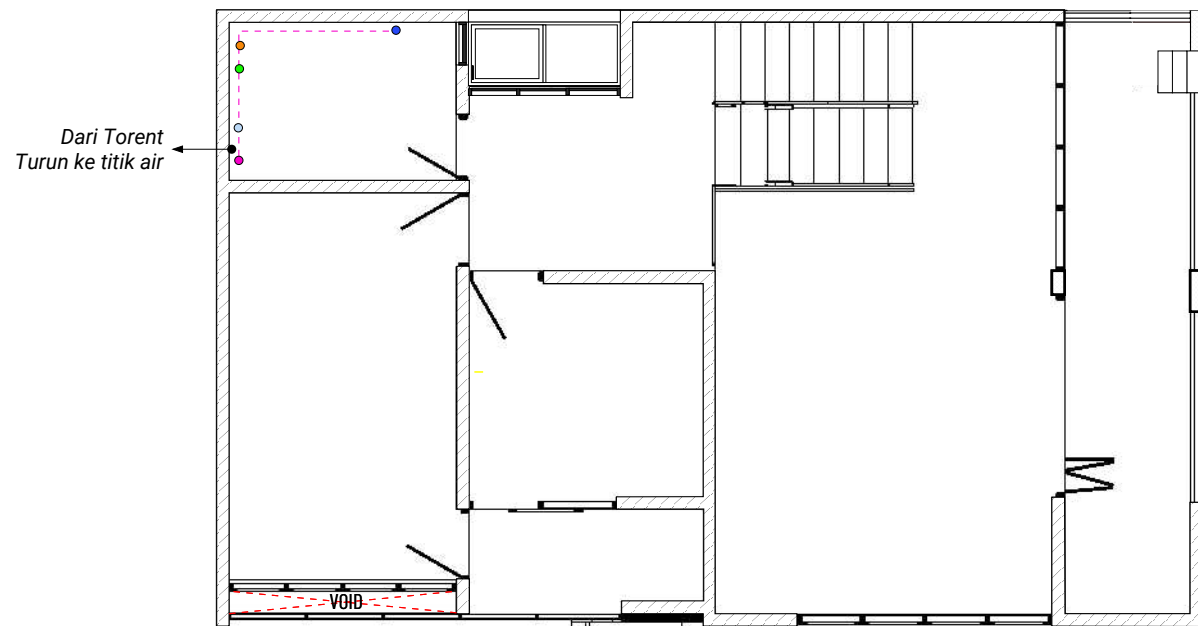
DENAH PLAFOND LANTAI 2 skala 1 : 100
