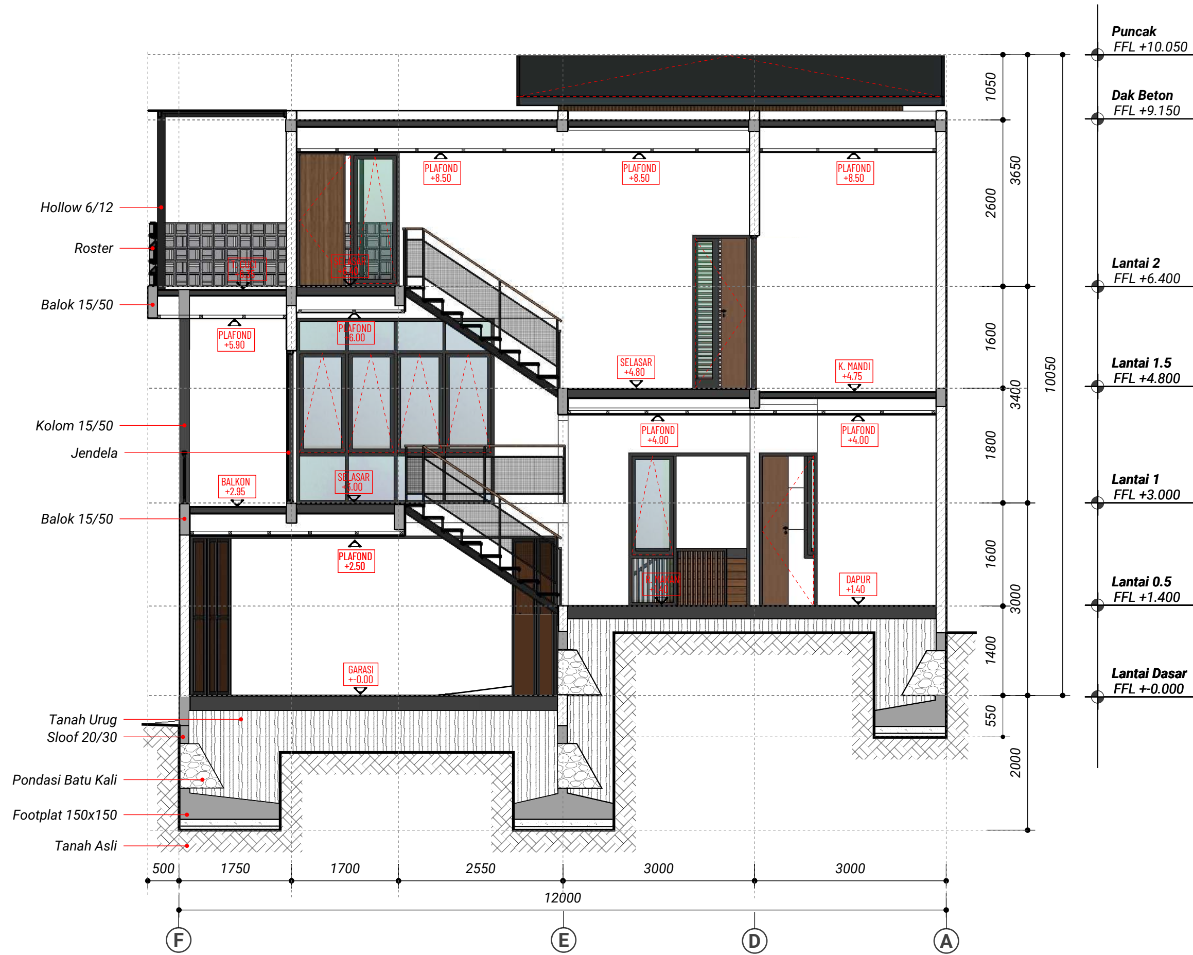
POTONGAN D-D skala 1 : 100
