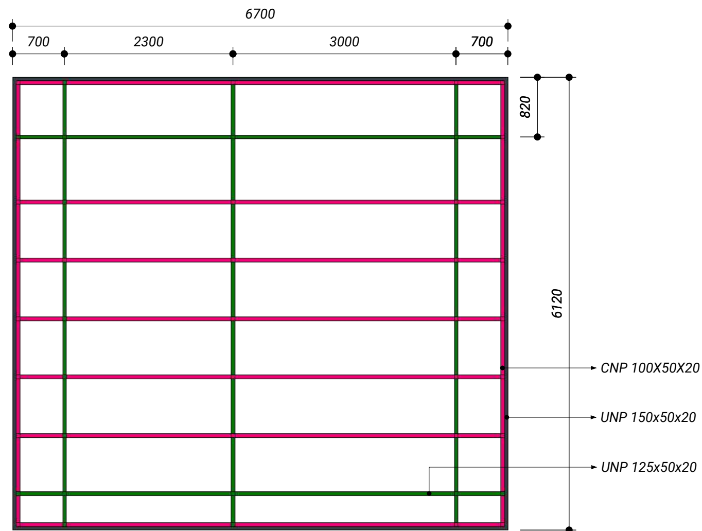
DENAH RANGKA ATAP skala 1 : 50
