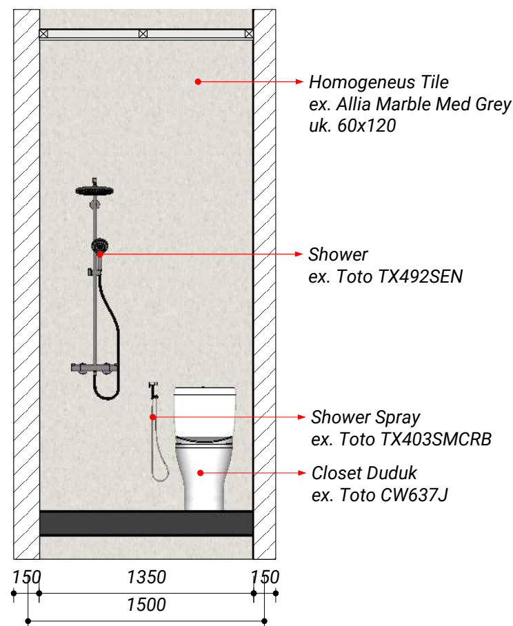
POTONGAN - A skala 1 : 50
