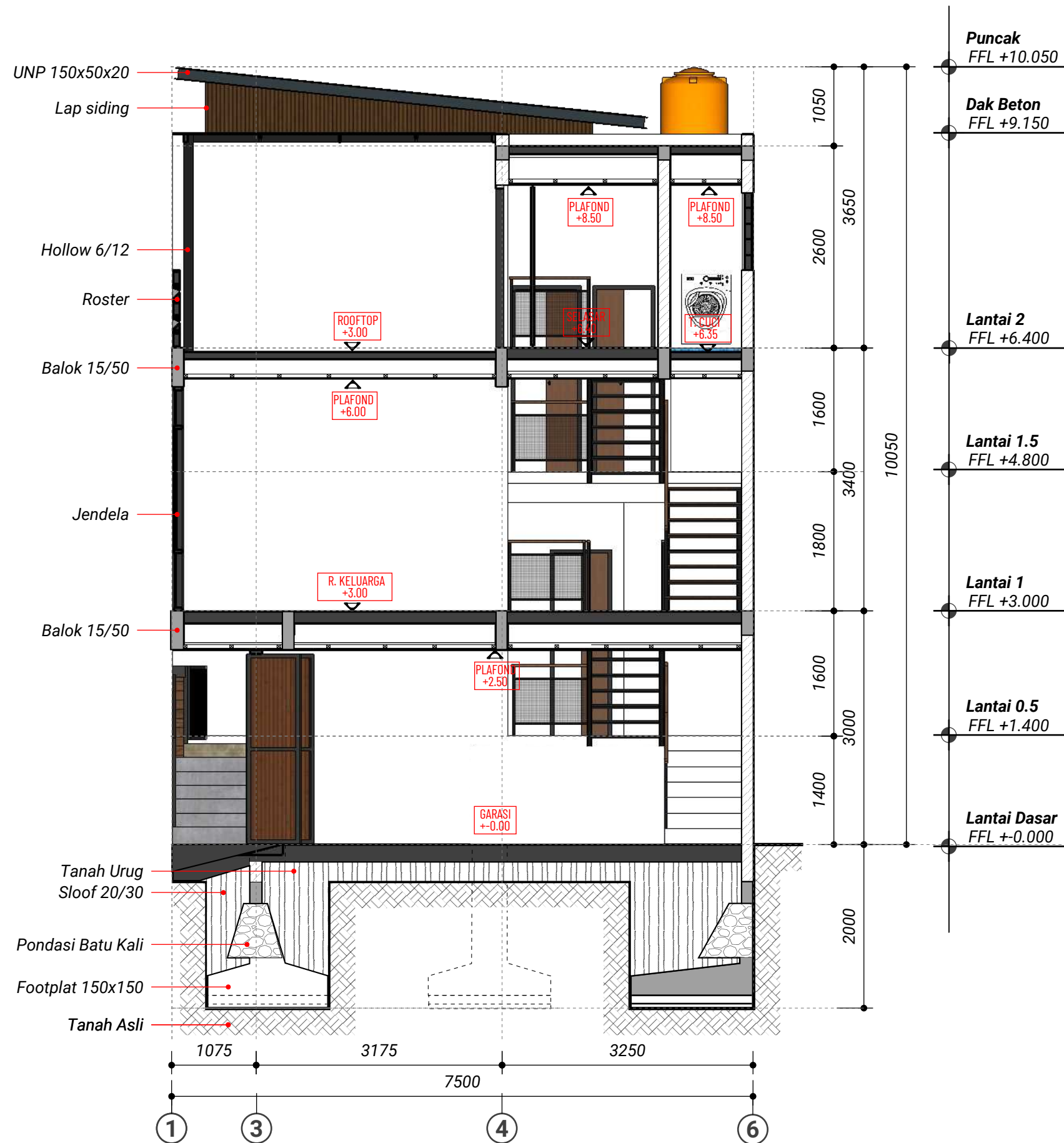
POTONGAN C-C skala 1 : 100
