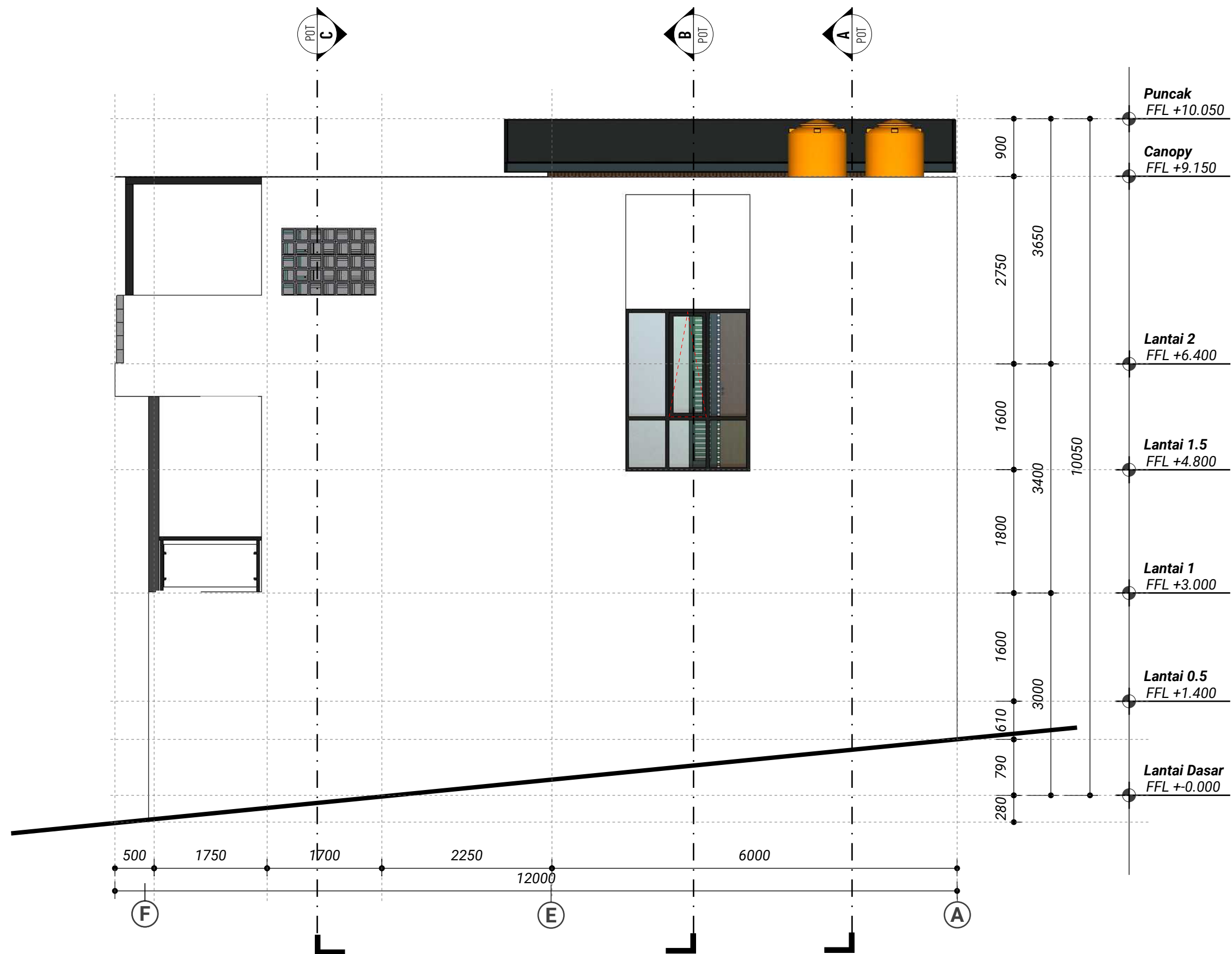
TAMPAK BELAKANG skala 1 : 100
