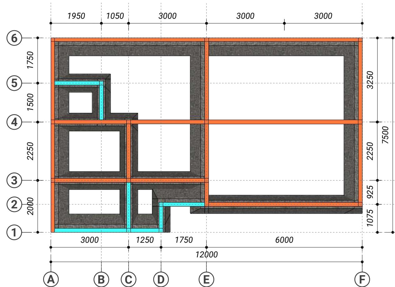
DENAH PONDASI skala 1 : 100
